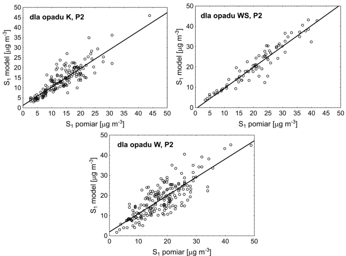
Rys 2. Porównanie zmierzonych i obliczonych stężeń PM_{10} po wystąpieniu krótkotrwałych opadów rozpatrywanych rodzajów.
